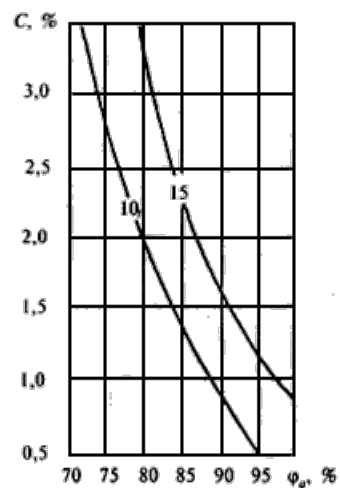
Рисунок Щ.3 - Изолинии сорбционного влагосодержания керамзитобетона \rho_0 = 1200 \text{ кг/м}^3 , содержащего хлорид магния, при изменении относительной влажности воздуха \phi_a , %, и массового солесодержания C , %
